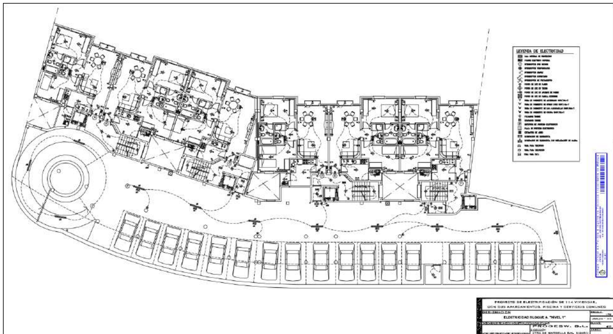
*Plano de instalación eléctrica de 114 viviendas
